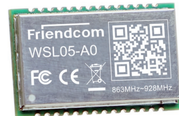
WSL05-868/915MHz
